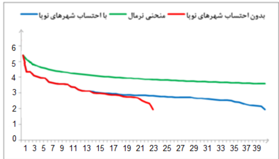
شکل ۴: تاثیر تبدیل روستا به شهر در سلسله مراتب شهری استان ۱۳۸۵
