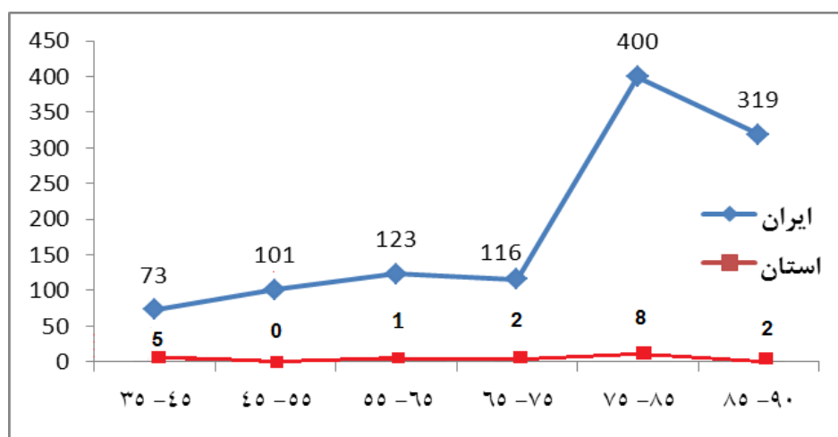
شکل ۲: تعداد روستاهای ارتقا یافته به شهر در ایران و استان
