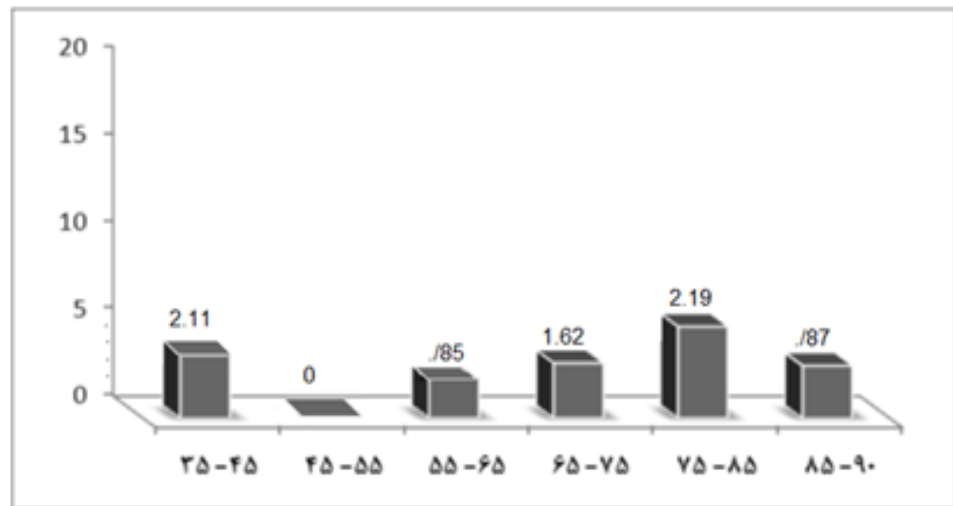
شکل ۳: درصد جمعیت اضافه شده به شبکه شهری استان از طریق تبدیل روستا به شهر
