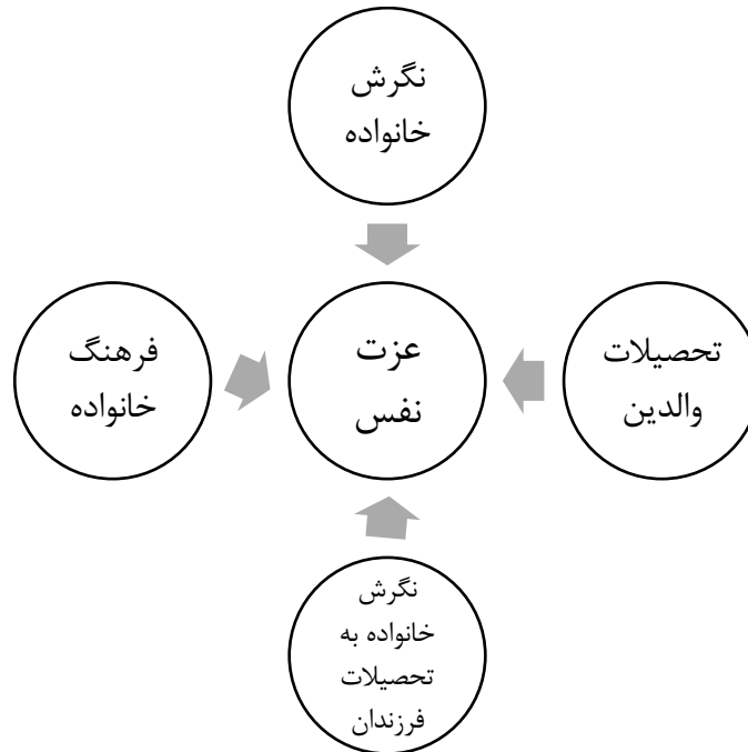
شکل ۱: مدل مفهومی
